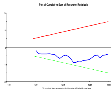
نمودار (۱): نتیجه استحکام مدل با استفاده از آزمون CUSUM
