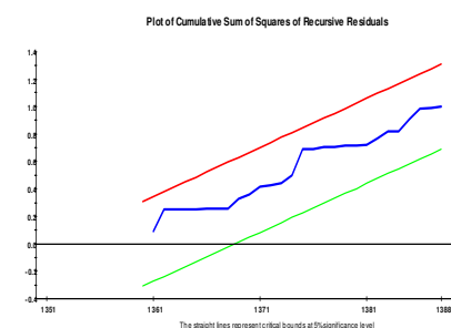
نمودار (۲): نتیجه استحکام مدل با استفاده از آزمون CUSUMSQ
